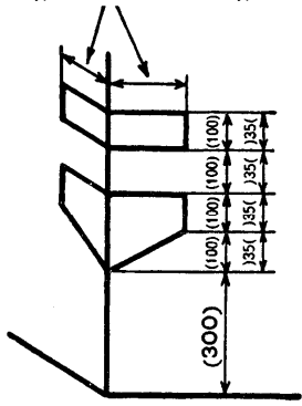
Figure 4 Largeur du montant d'angle
